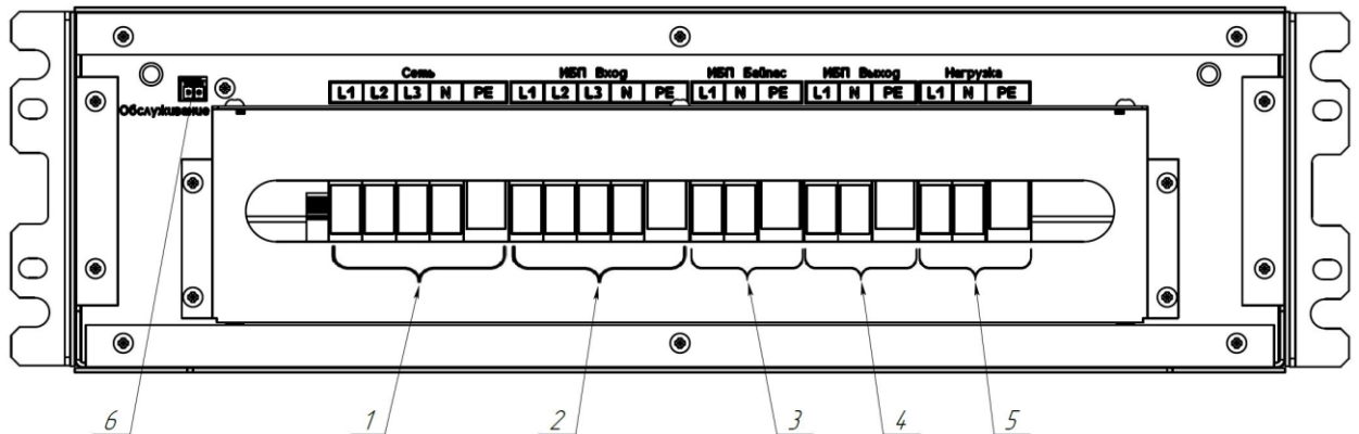
Рисунок 2 Габаритно-присоединительные размеры ББ. Вид сзади.
