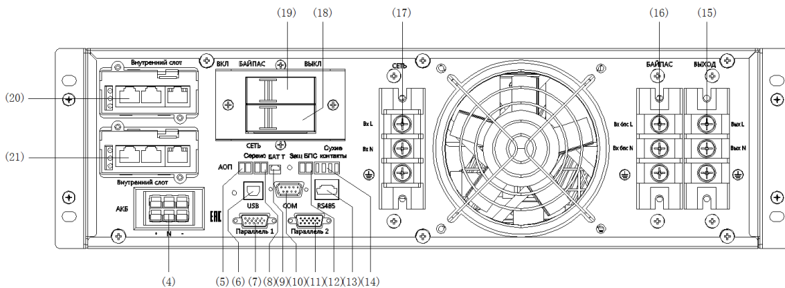
Вид сзади
