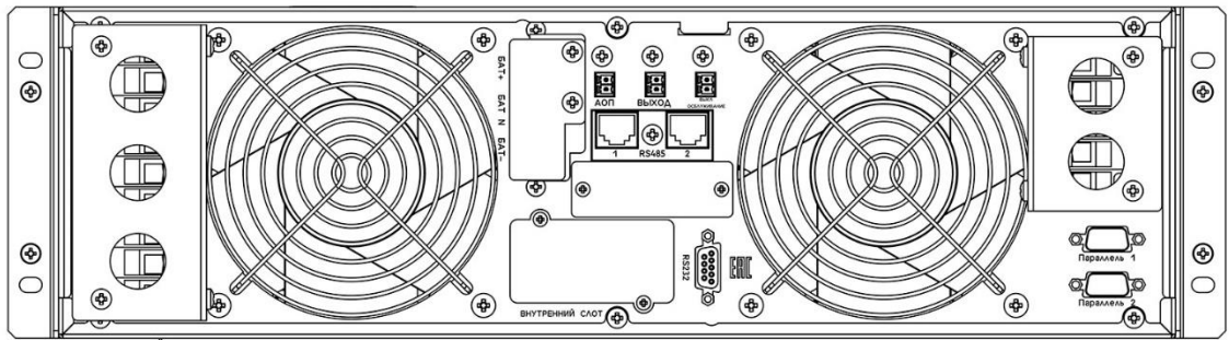
Вид сзади
