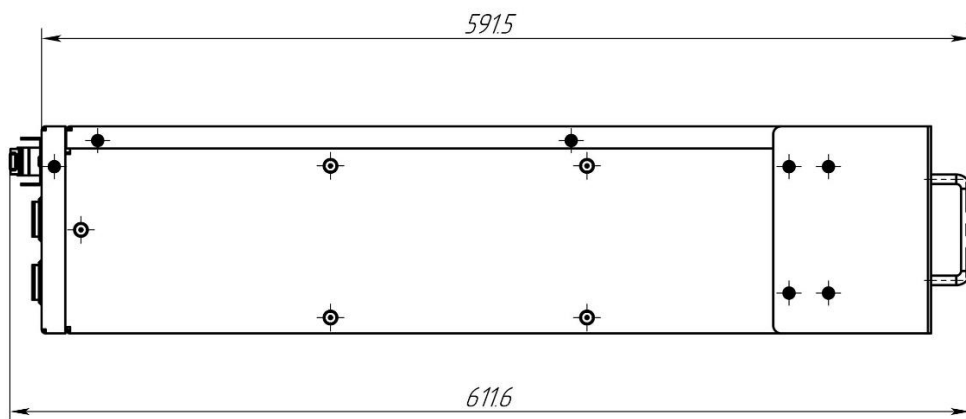
Вид сбоку
