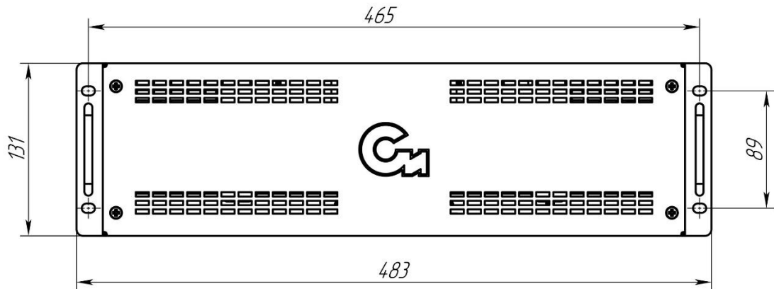
Вид спереди
