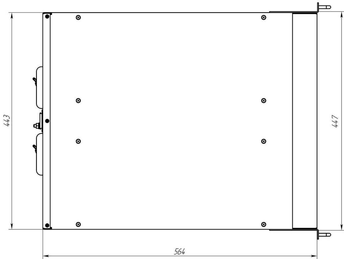
Вид сверху
