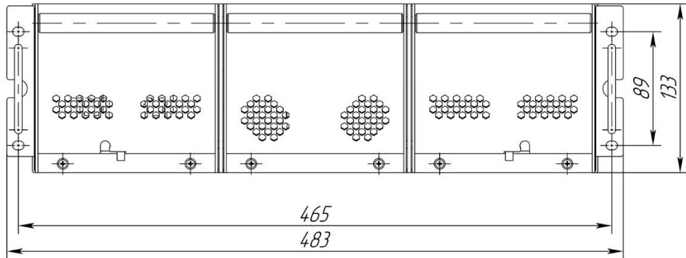
Вид спереди
