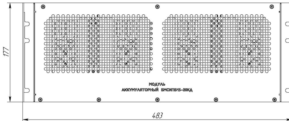
Вид спереди
