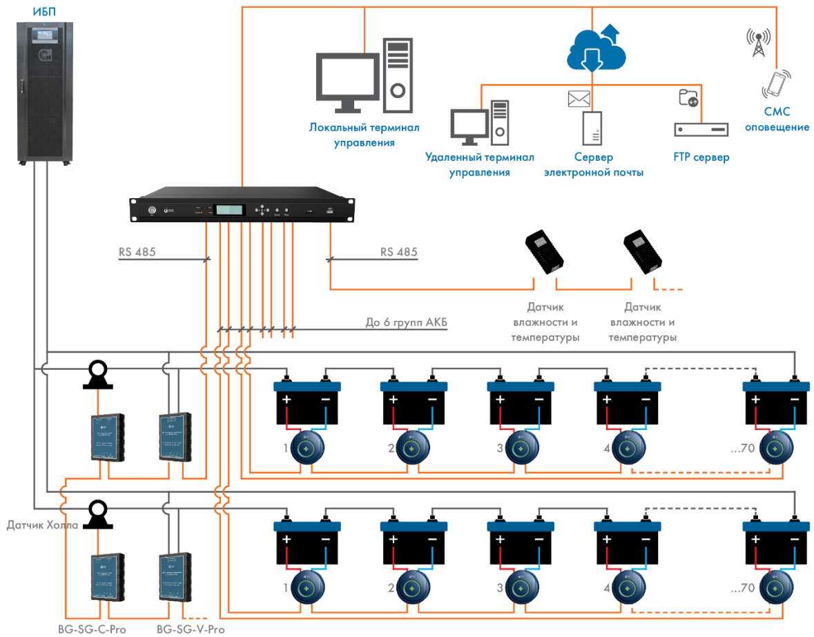
Схема построения системы мониторинга на контроллере BG-BMS-Rack-6G-70
